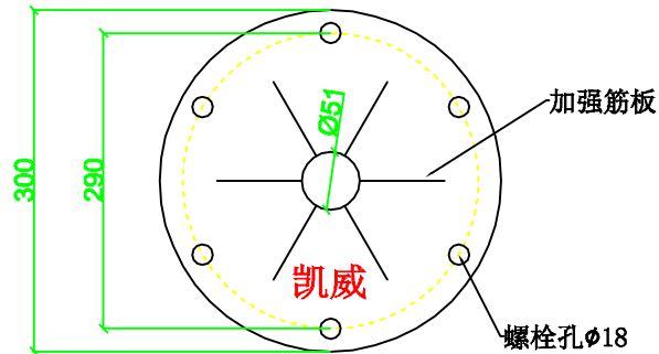
法兰尺寸图
